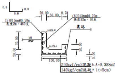
標準断面圖 S=1/50 U=m L=92m
