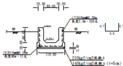
標準断面圖 S=1/50 U=m L=46m
