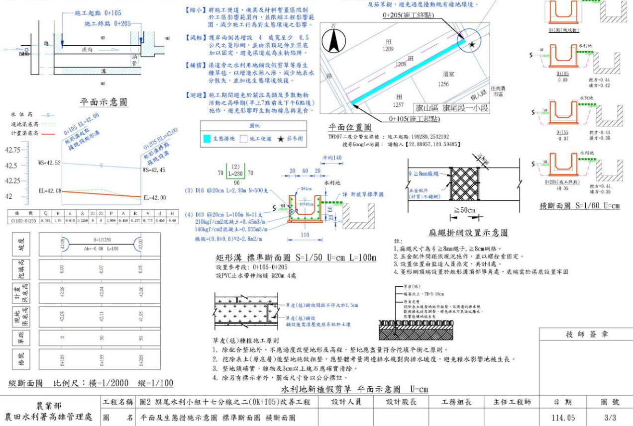
圖2 旗尾水利小組十七分線之二(0K+105)改善工程(矩形溝100m)
